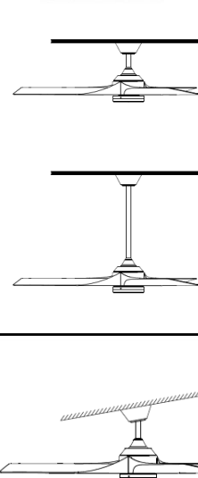
Instalación de varilla
