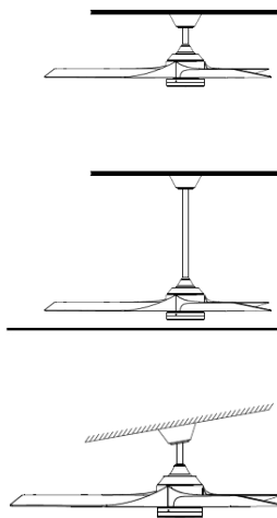
Installation de la tige de suspension
